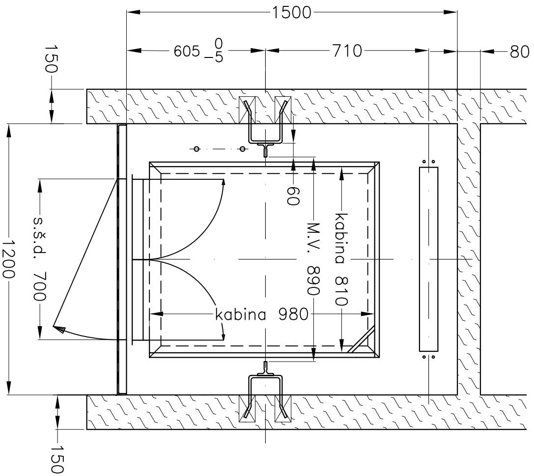
PŮVODNÍ KONSTRUKCE
