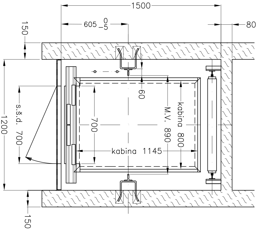
PO REKONSTRUKCI
